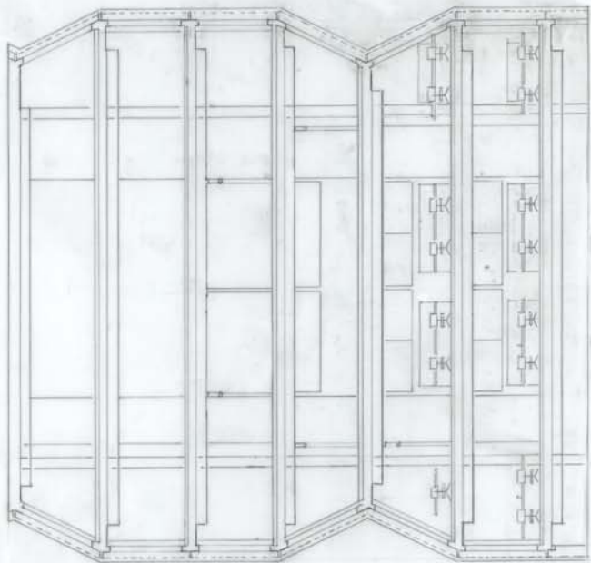
TYPSEKTION 1 100
